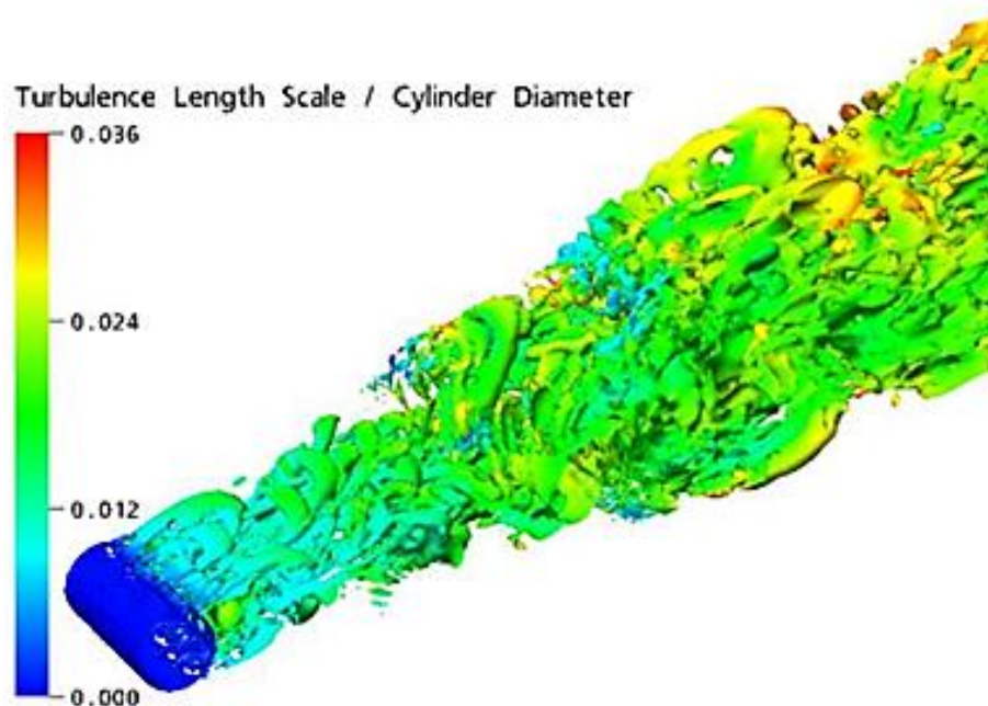
Turbulentes Längenmaß der Strömung im Nachlauf eines Zylinders
